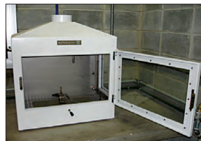
Figura 44: Determinação da ignitabilidade dos materiais
