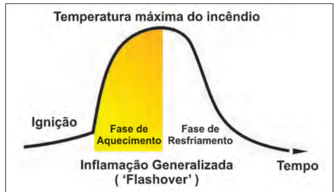
Figura 20: Curva temperatura - tempo de um incêndio
