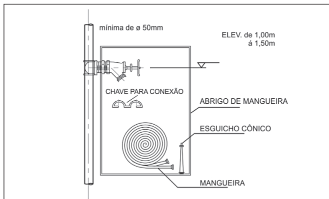
Figura 63: Detalhe de hidrante
